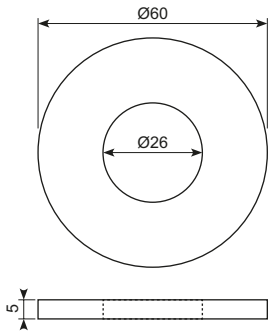
M24-skive til gummibuffer M24 washer for rubber buffer
